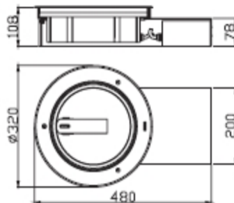
B: 分体式尺寸图
